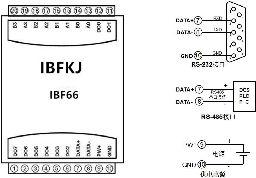
图 3 IBF66 模块接线图
