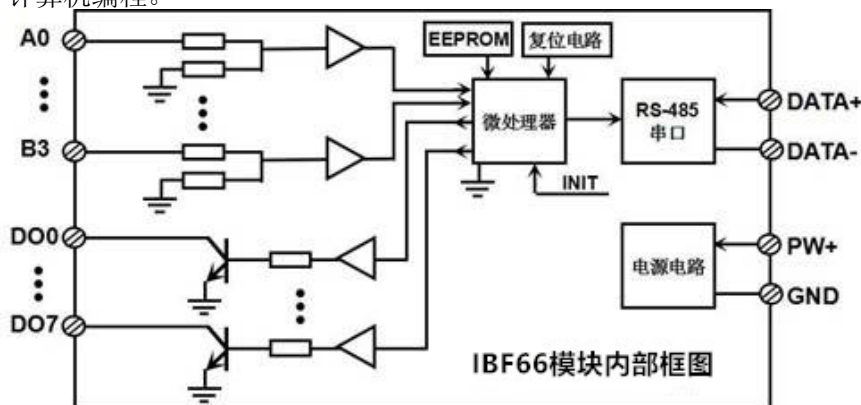
图2 IBF66 模块内部框图
