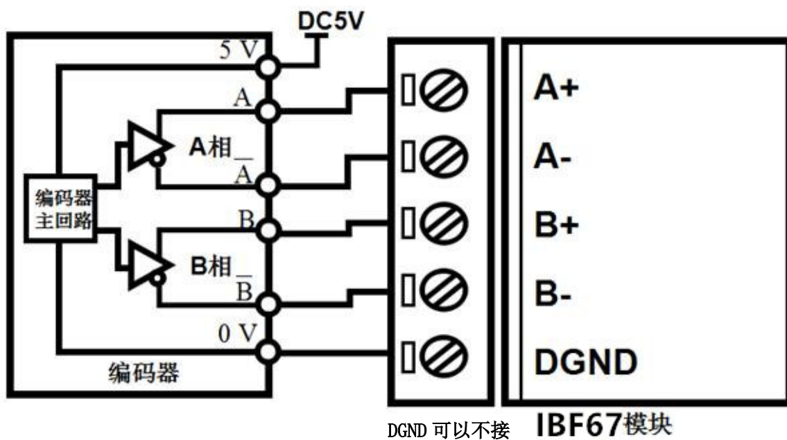
图3 IBF67 模块接线图
