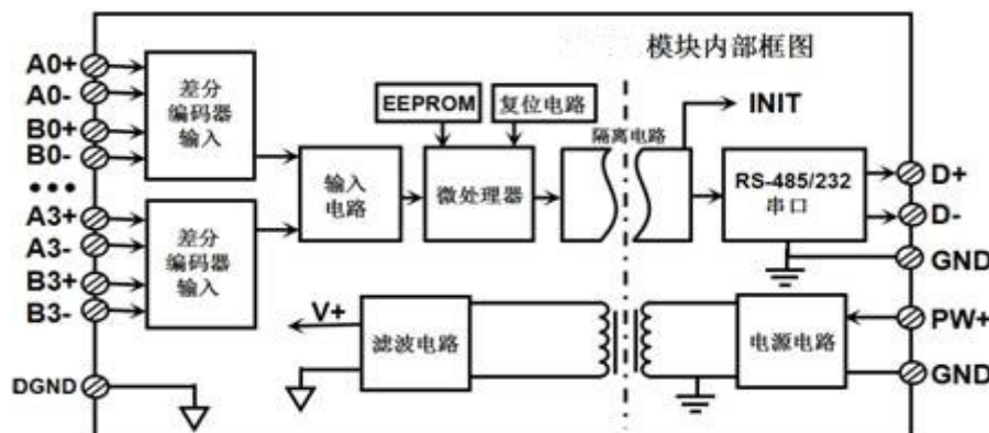
图2 IBF67 模块内部框图
