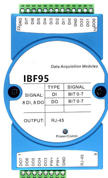
图1 IBF95 模块外观图
