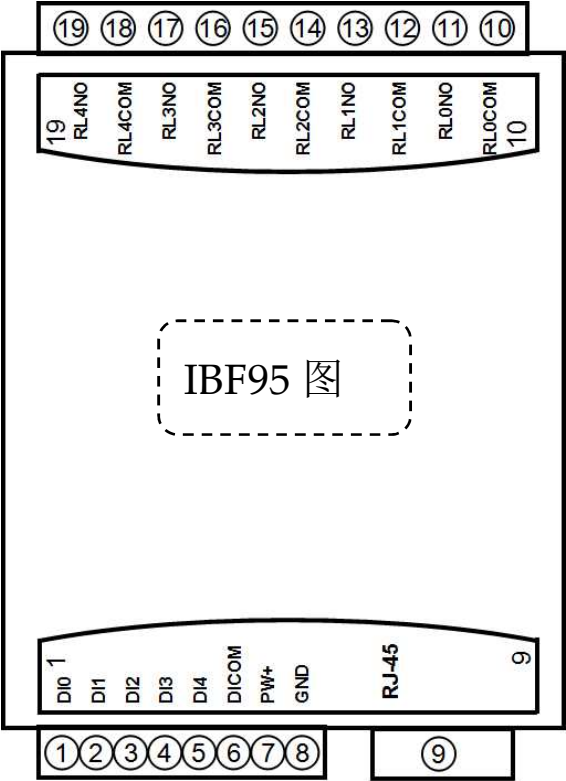
图 5 IBF95 模块接线图
