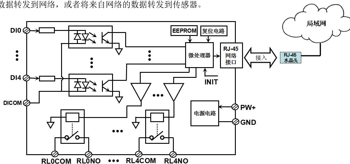
图2 IBF95 模块内部框图
